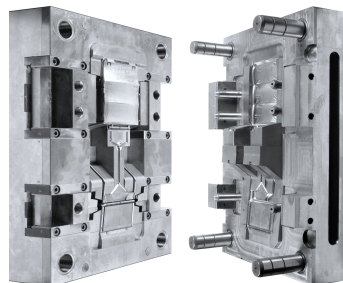
Spritzgießform "Wrangler-Jeep" von Weiss Umformwerkzeuge
